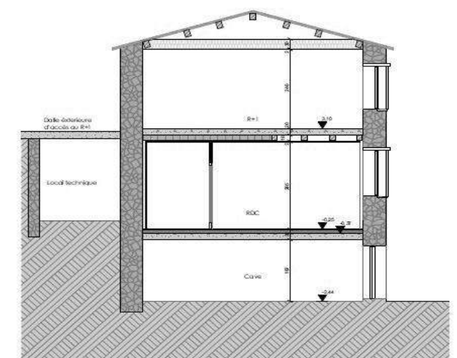
COUPE AA Projet
