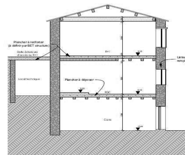
COUPE AA Existant
