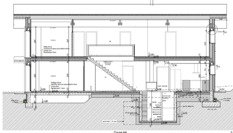
Coupe AA
