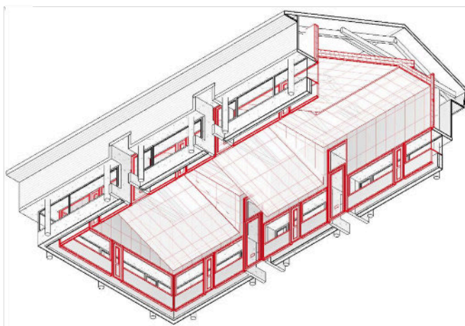
Axonométrie vue de dessous
