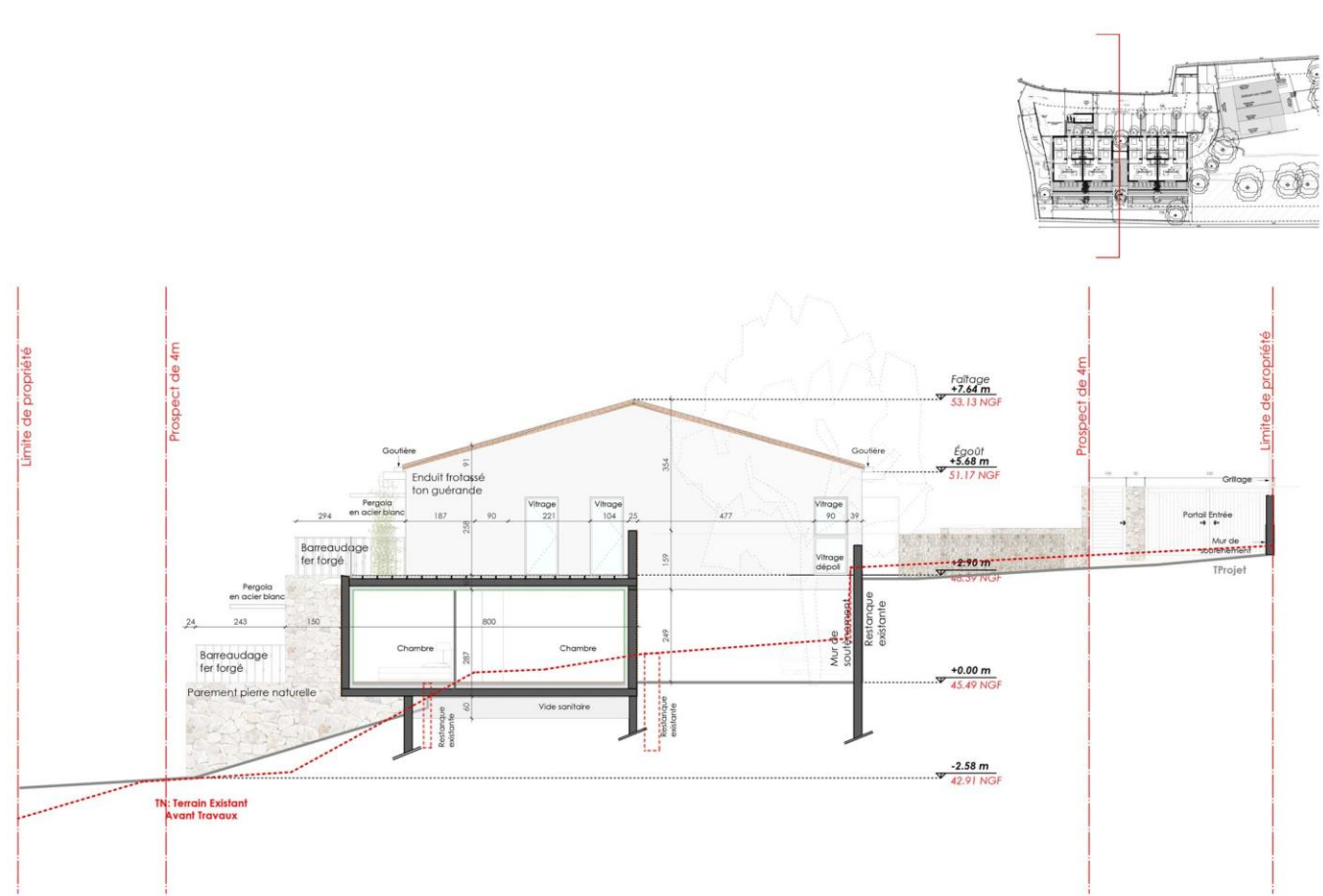
Coupe BB'
