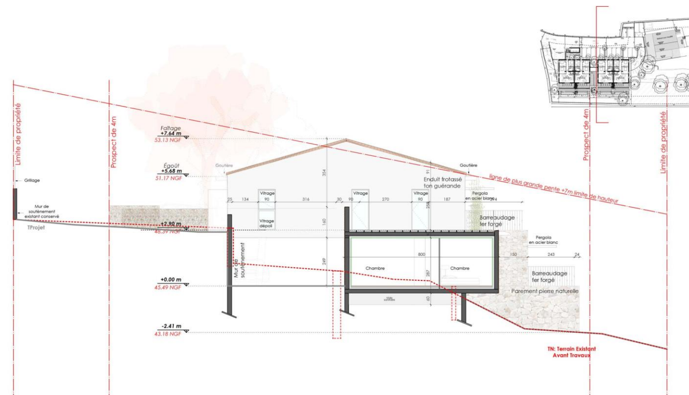
Coupe DD'
