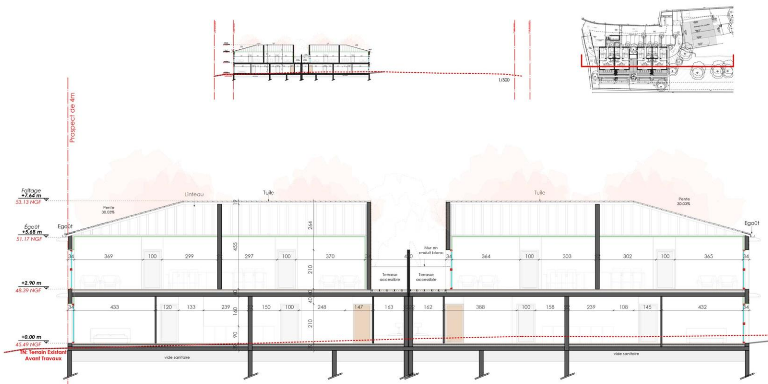
Coupe AA'
