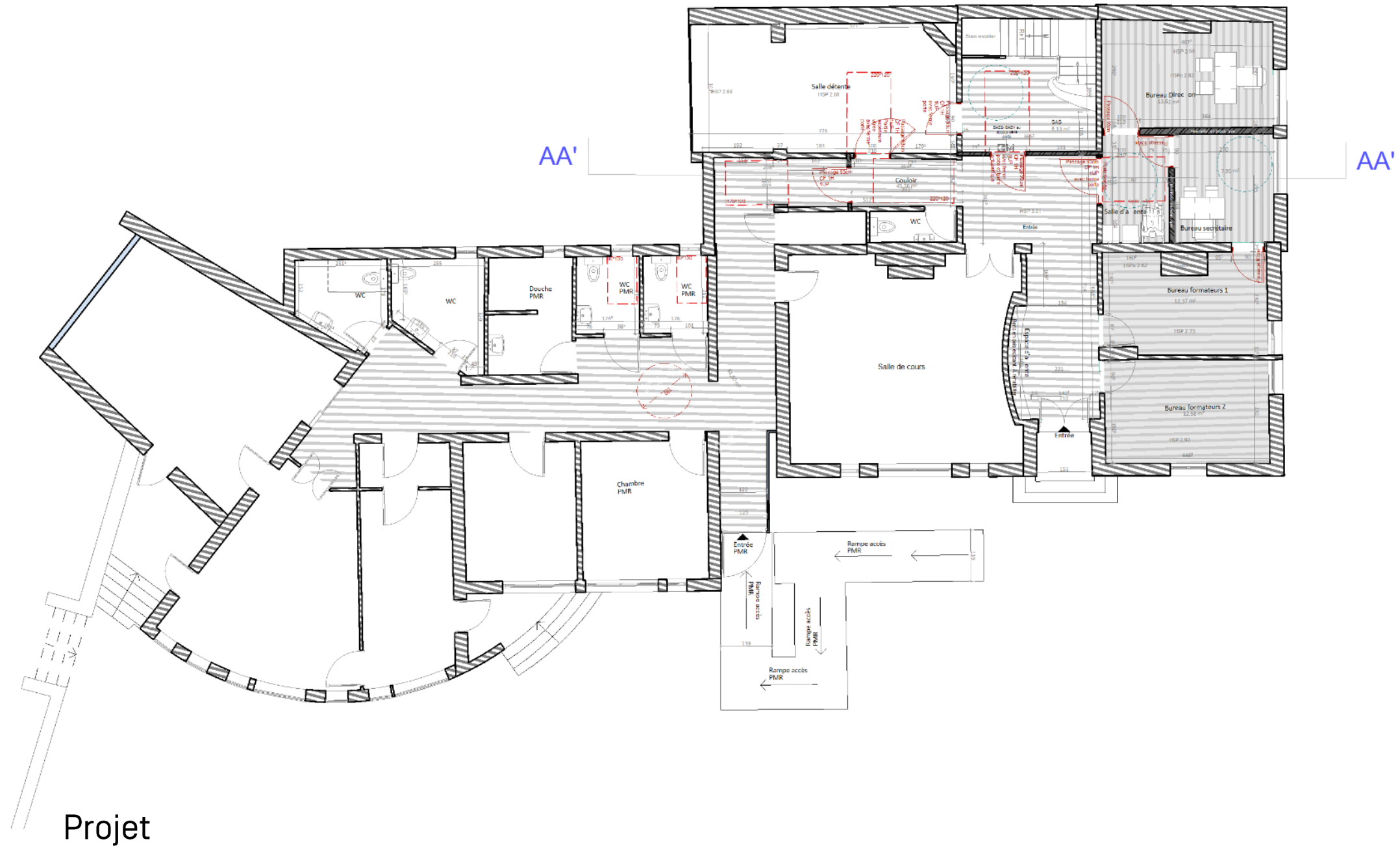
Avant-projet
