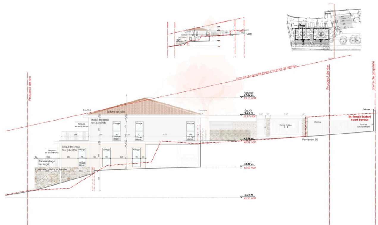
Façade est
