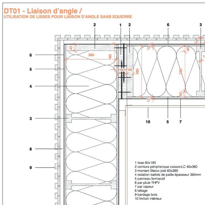
Détail sur une liaison d'angle
