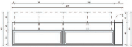
Coupe BB'
