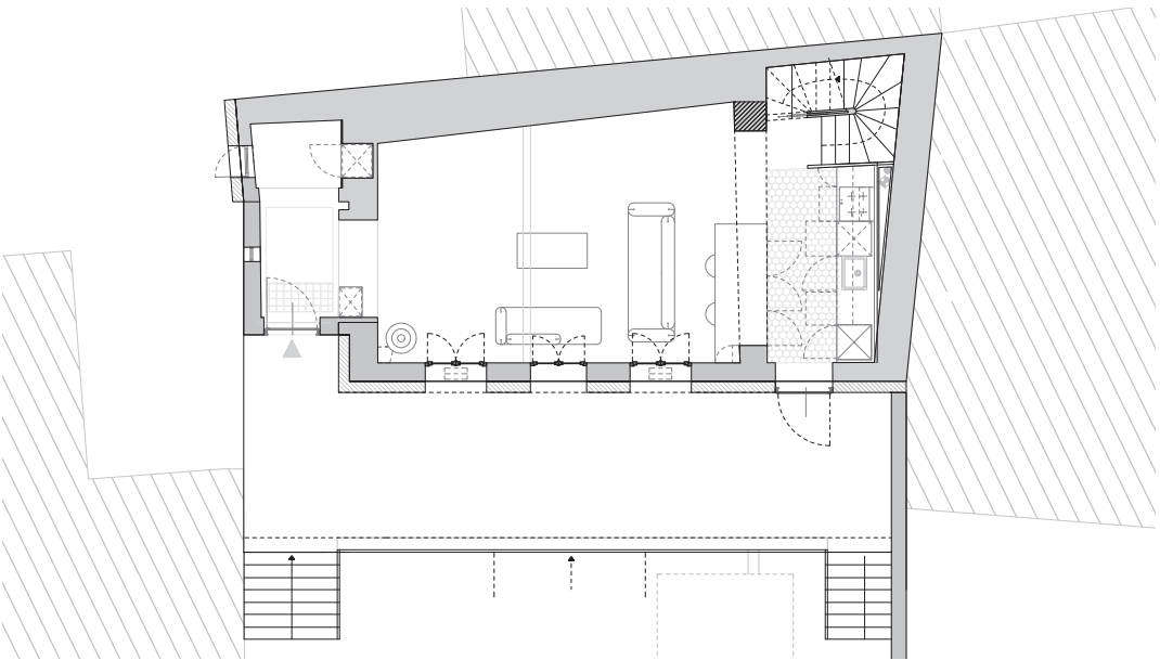
Plan RDC
