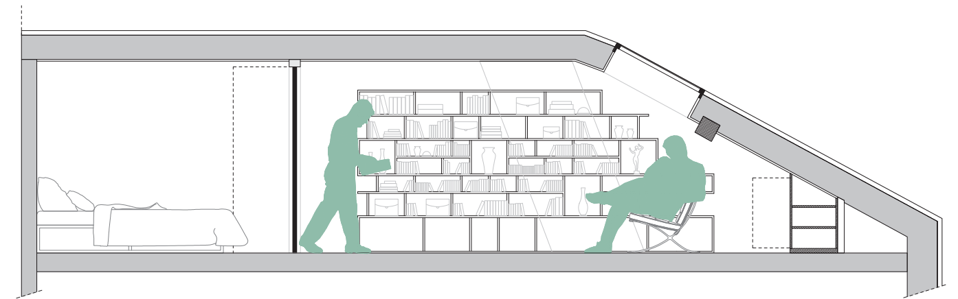
Coupe BB'
