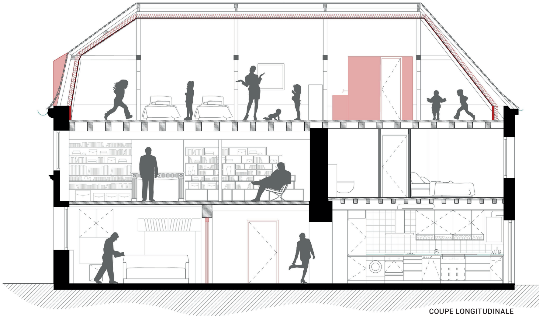
COUPE LONGITUDINALE
