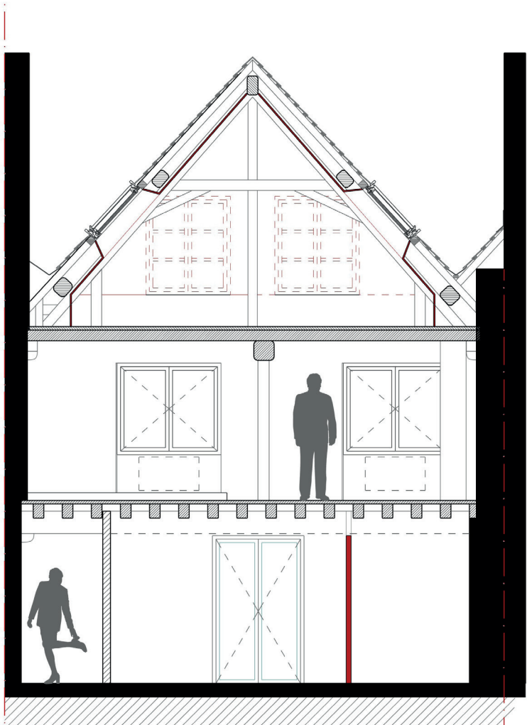
COUPE TRANSVERSALE
