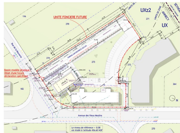
Plan masse - 1.500
