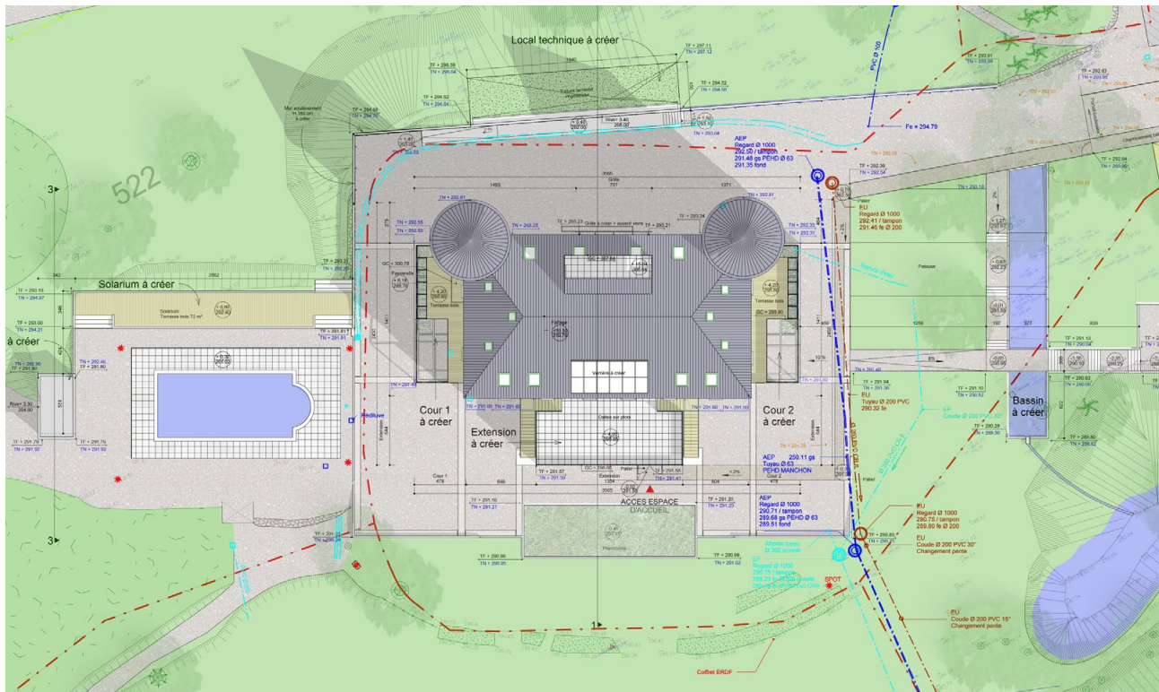
Plan masse aménagement - 1.200
