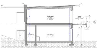
Coupe BB - 1.50
