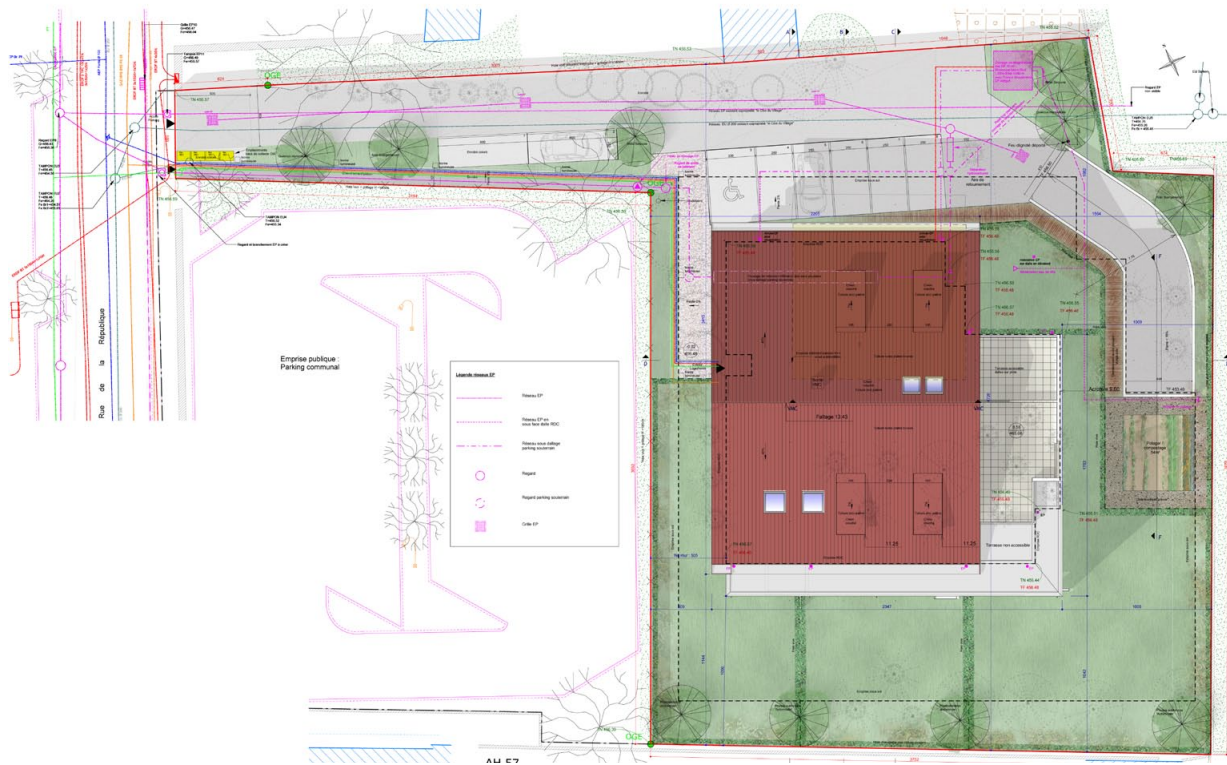
Plan Masse - 1.100
