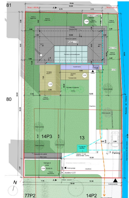
Plan masse - 1.100
