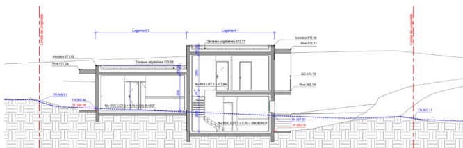
Coupe BB - 1.100
