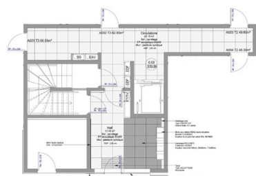
Détails Hall d'entrée - 1.50
