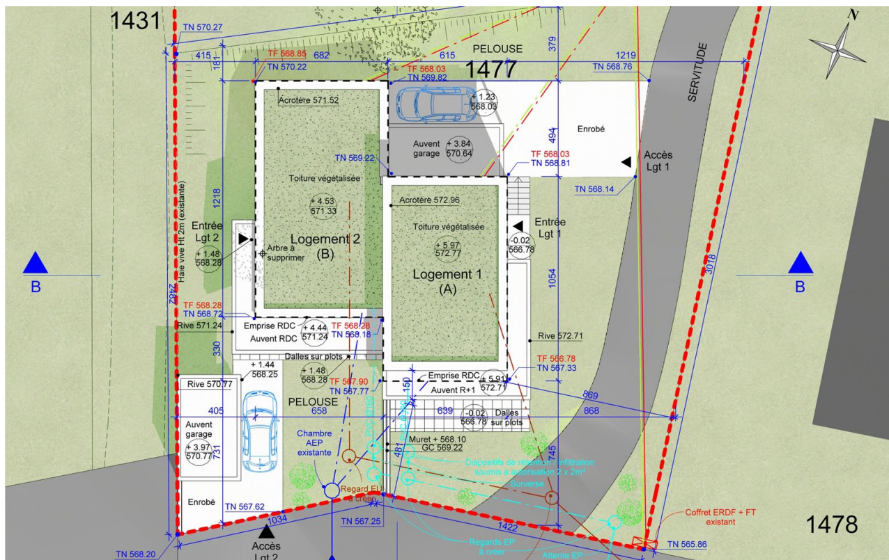
Plan masse - 1.200
