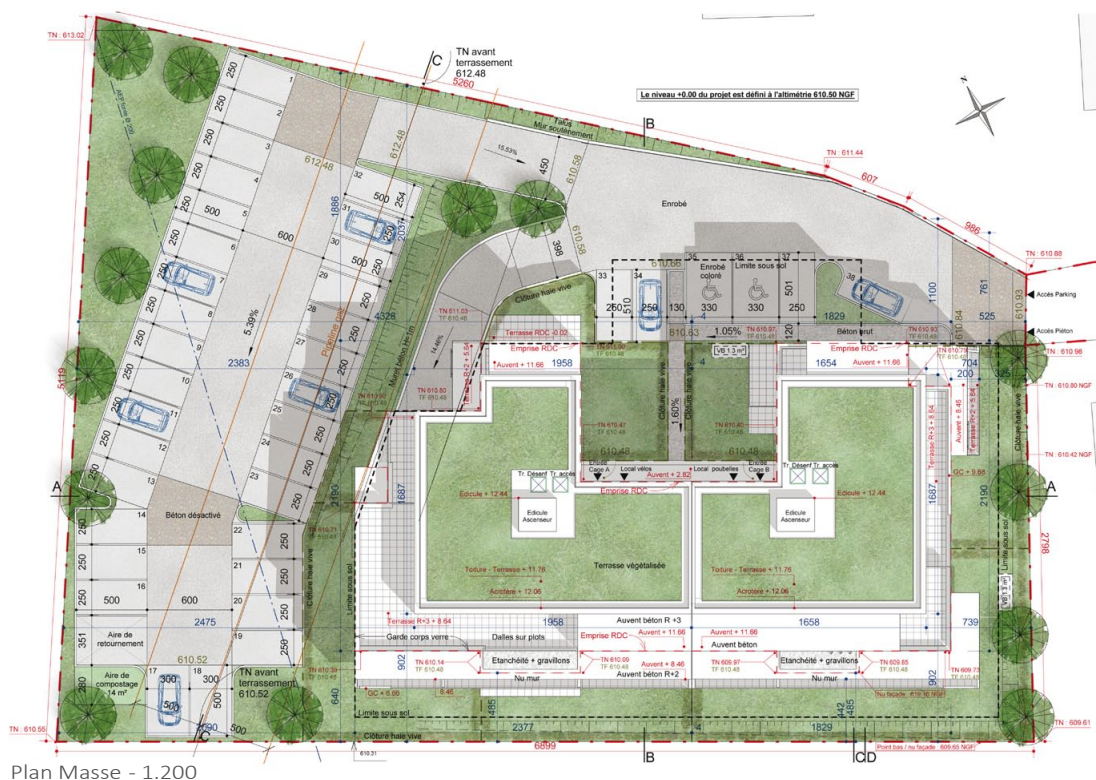
Plan Masse - 1.200
