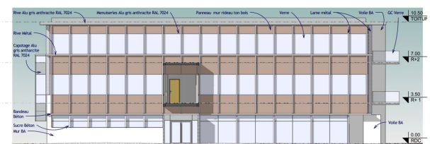
Façade Sud Est - 1.200
