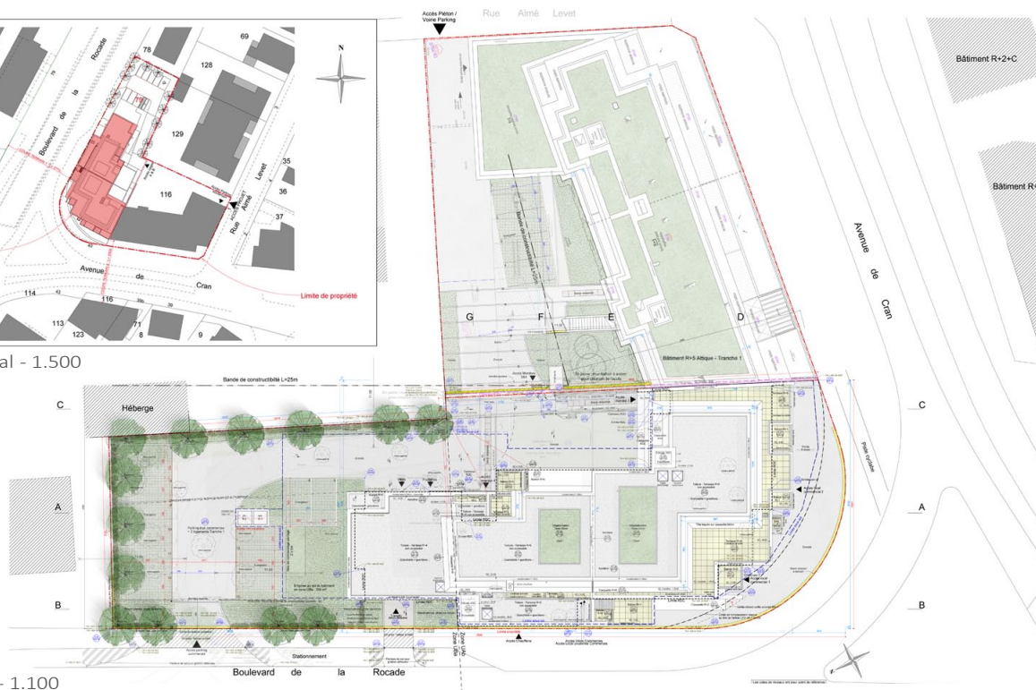
Plan Masse - 1.100
