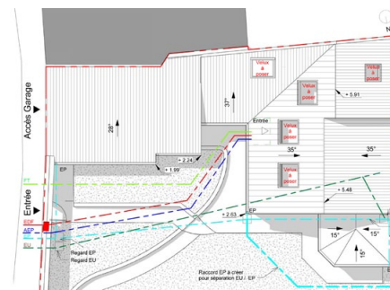
Plan masse - 1.200
