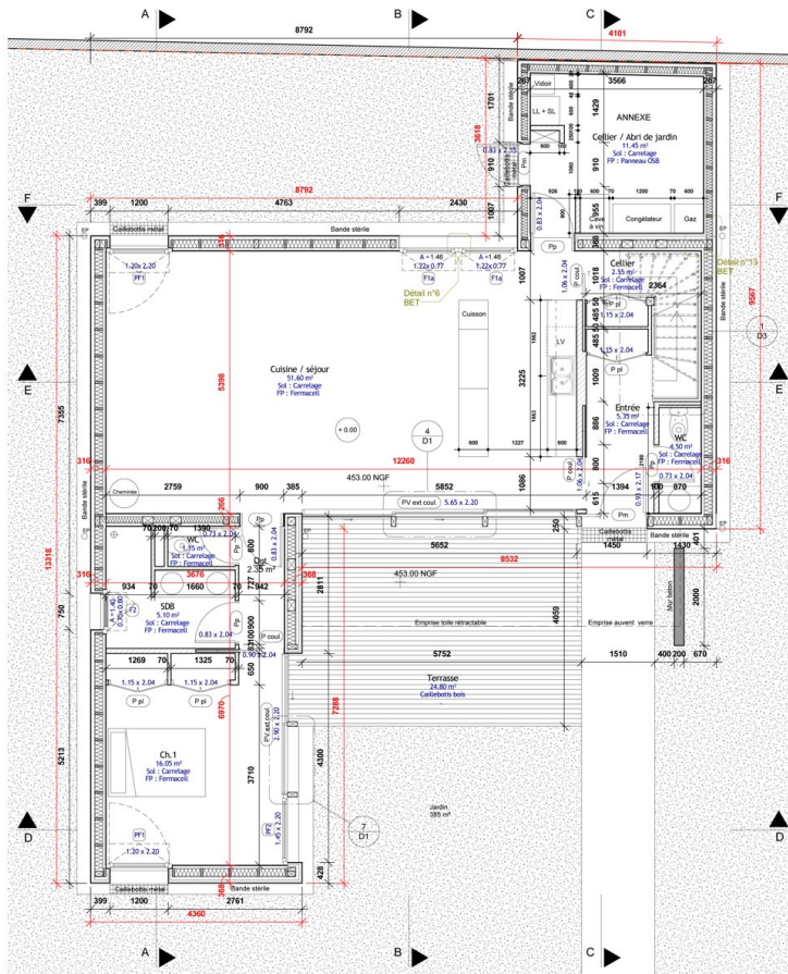
Plan RDC - 1.50
