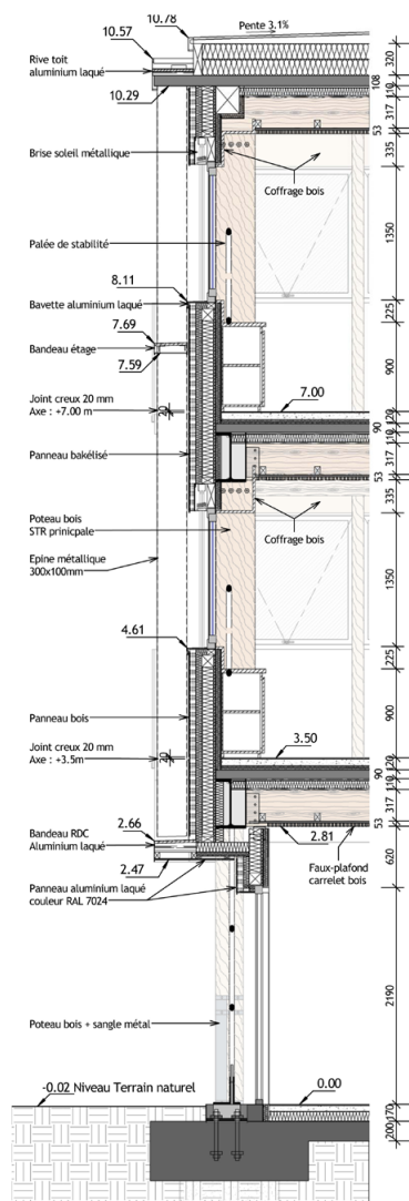
Coupe détail - 1.30
