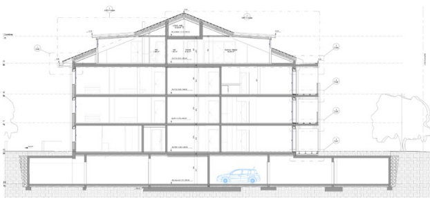
Coupe BB - 1.100
