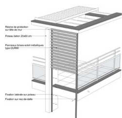
Détail brise soleil
