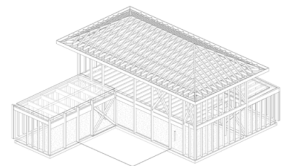
Axonométrie structure bois
