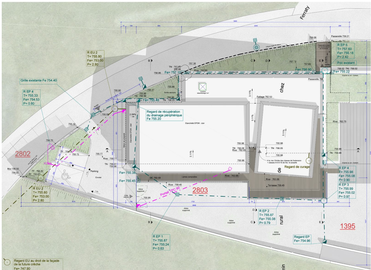
Plan Masse - 1.100
