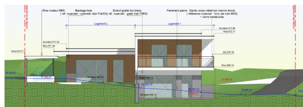
Façade Sud - 1.100
