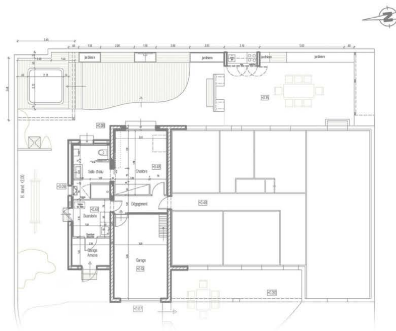
Extension d'une villa et aménagement du jardin, avec création d'espaces extérieurs de relaxation - Villa CG - Nissan lez Enserune - 2008
