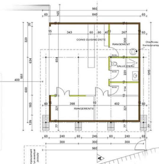
Aménagement des espaces extérieurs d'un Domaine, avec création d'une piscine haut standing et de son pool house, construction d'un cour de tennis, création d'espace de détente, de réception - Laure Minervois - 2001 / 2011 Réalisation avec Agence AD
