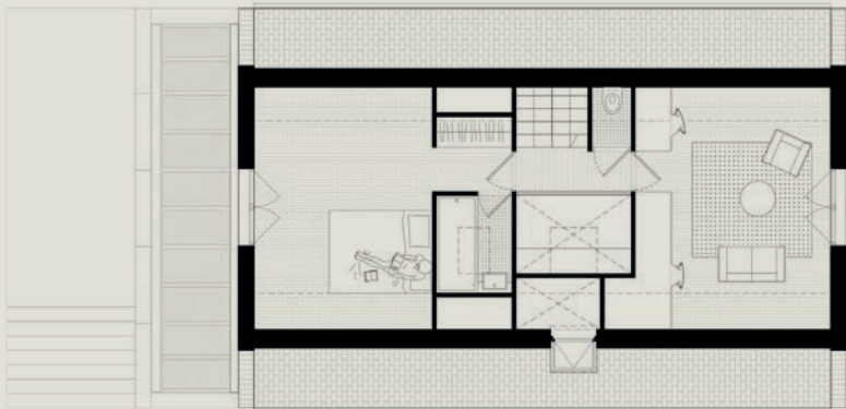
Plan R+2
