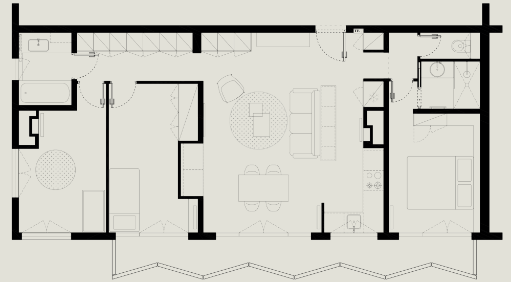
Plan projet
