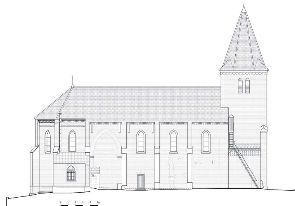
Elévation sud
