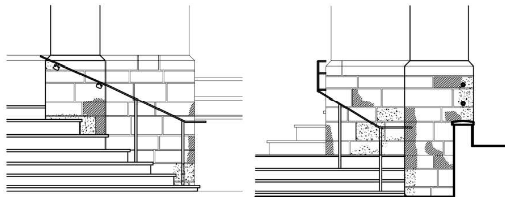
Façade ouest
