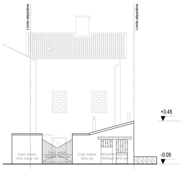
façade Sud existant
