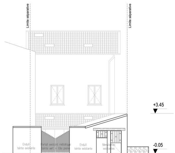
façade Sud projet
