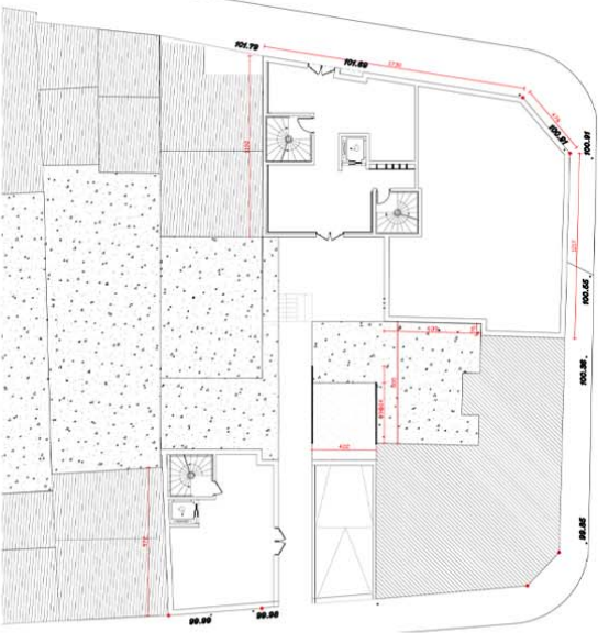
plan RDC
