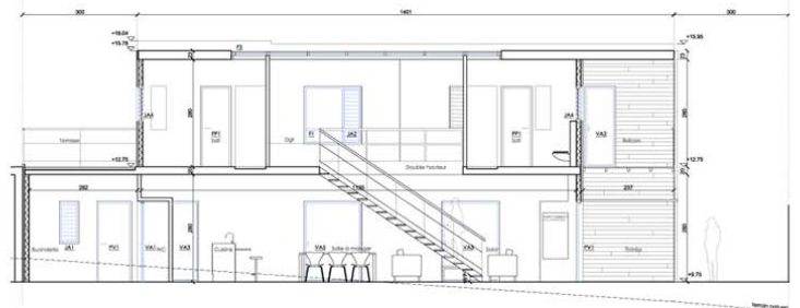
coupe longitudinale 88
