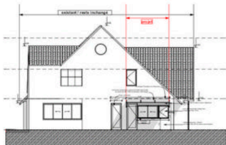
Facade Nord-Est, Projeté
