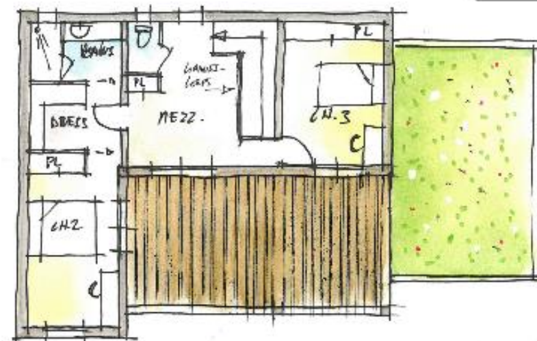
NIVEAU 1 1/100°
