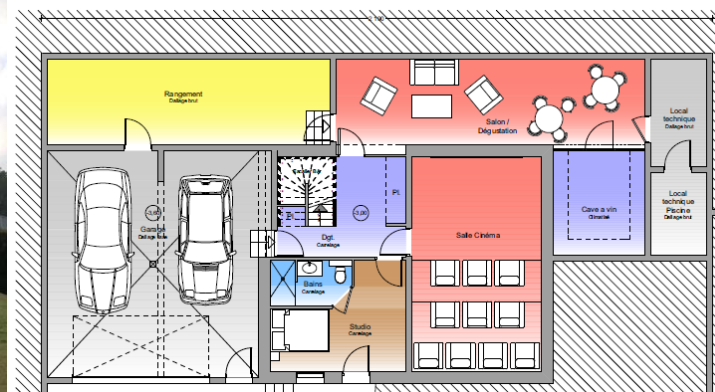
Sous-sol
