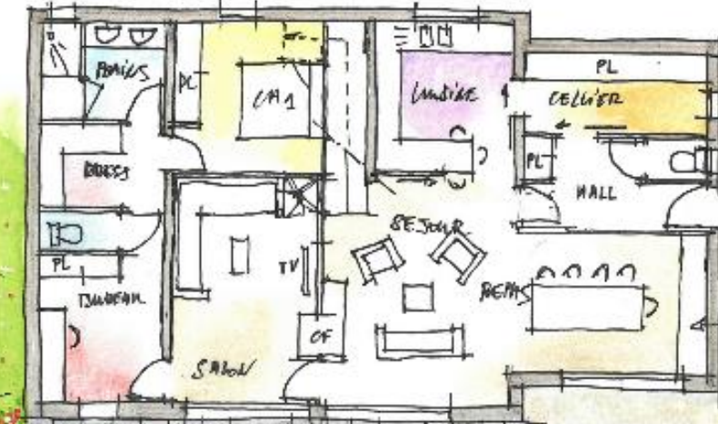
NIVEAU RDC 1/100°
