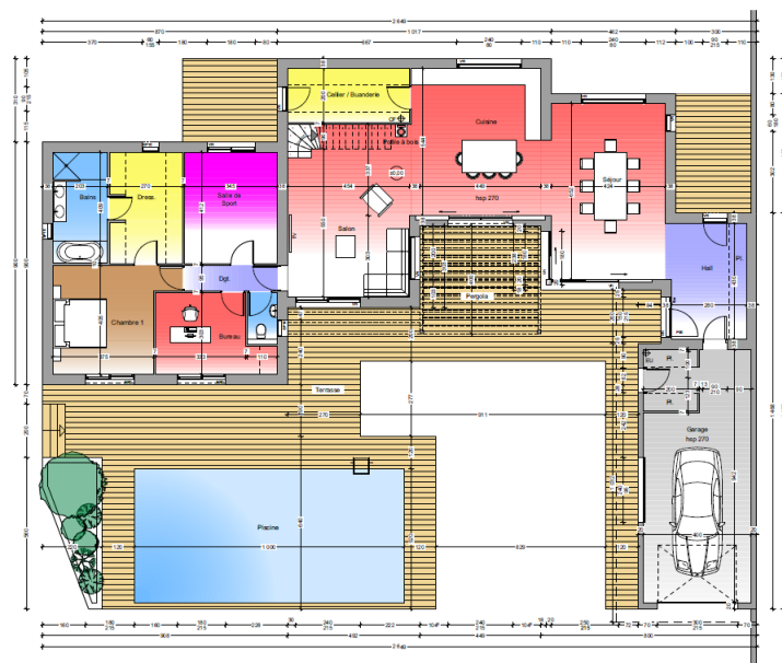
Rez-de-Chaussée
