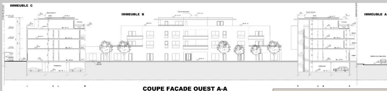
COUPE FAÇADE OUEST A-A
